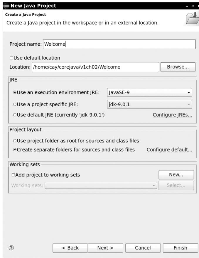
Рис. 2.6. Настройка проекта в Eclipse
